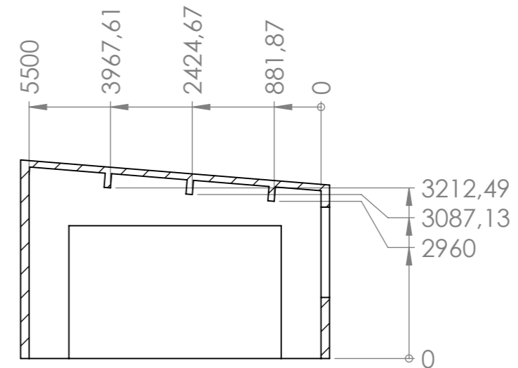
PRZEKRÓJ C-C
